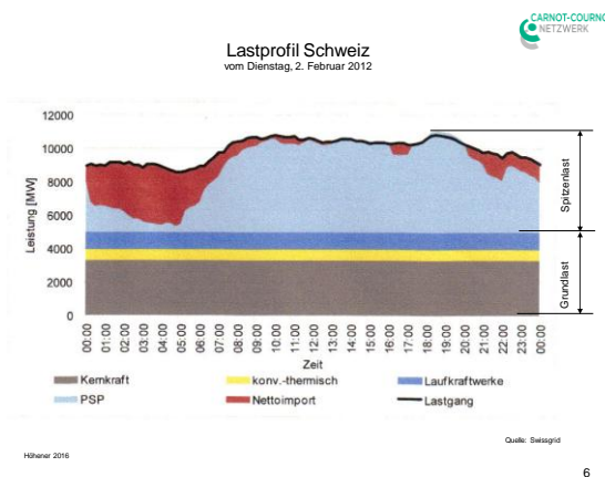
Abbildung 5 Typisches Lastprofil Schweiz
