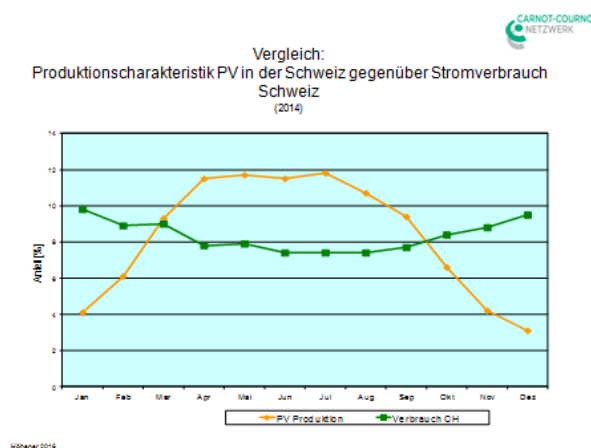
Abbildung 6 Jahresproduktions-Verlauf PV gegenüber Verbrauch
