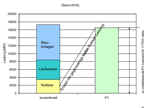
Vergleich der zu installierenden PV Leistung zur gegewärtigen Leistung konventioneller Anlagen.
