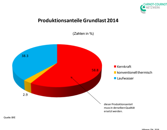
Abbildung 4 Produktions-Anteile Grundlast
