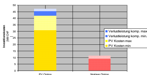
Kostenvergleich PV- System Option für 11.0TWh Jahresproduktion in Grundlastqualität gegenüber KKW Produktion gleicher Grössenordnung nicht berücksichtigt sind Systemkosten für Pumpspeicherung und allfällige Kosten für Land
